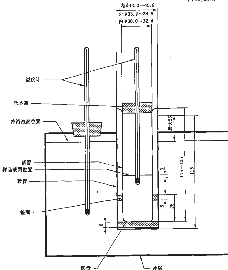
图1 倾点测定仪
